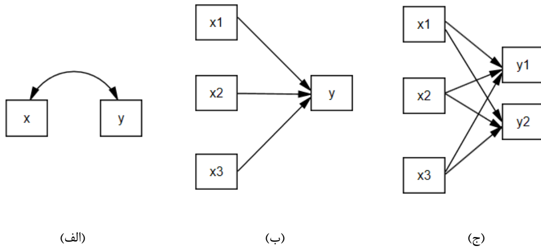
شکل ۲. الگوی شماتیک همبستگی، رگرسیون خطی و تحلیل چند متغیره
